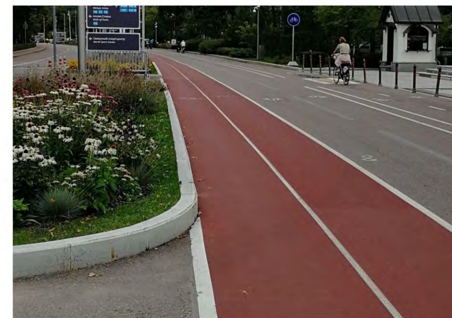
ХОРОШО. Мощение велосипедной полосы выполнено из цветного асфальтобетона
