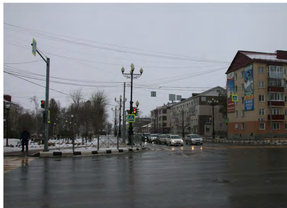
ПЛОХО. Излишнее количество светильников, воздушная прокладка проводов
